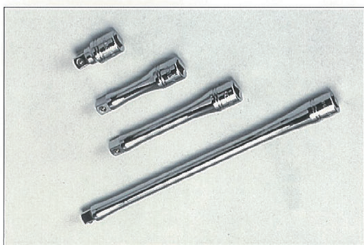
ネブロスシリーズ6.3sq.エクステンションバー ¥1,060~1,870 京都機械工具株式会社 オーディンデザイン株式会社 代表取締役井川喜市
